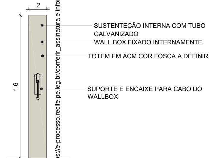
ELEV. LATERAL 02
