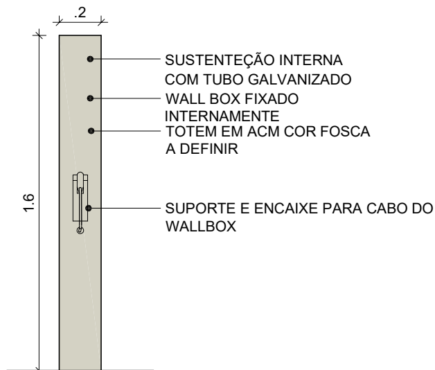
ELEV. LATERAL 01
