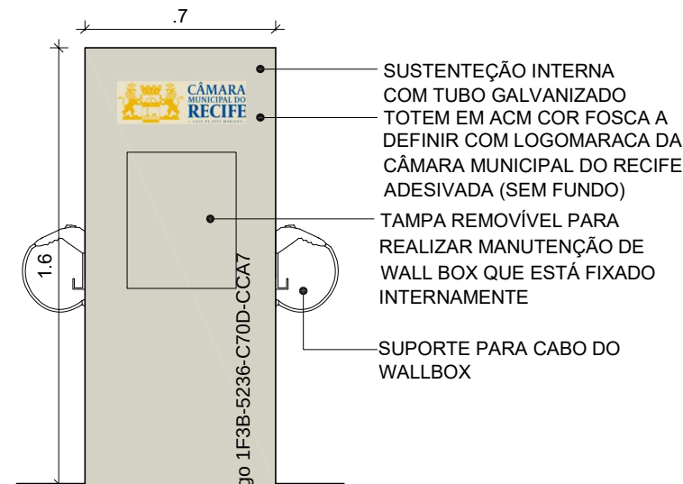
ELEVAÇÃO POSTERIOR
