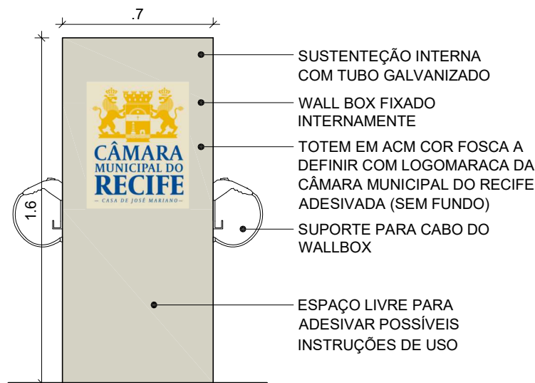
ELEVAÇÃO FRONTAL
